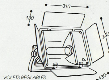
VOILETS RÉGLABLES
