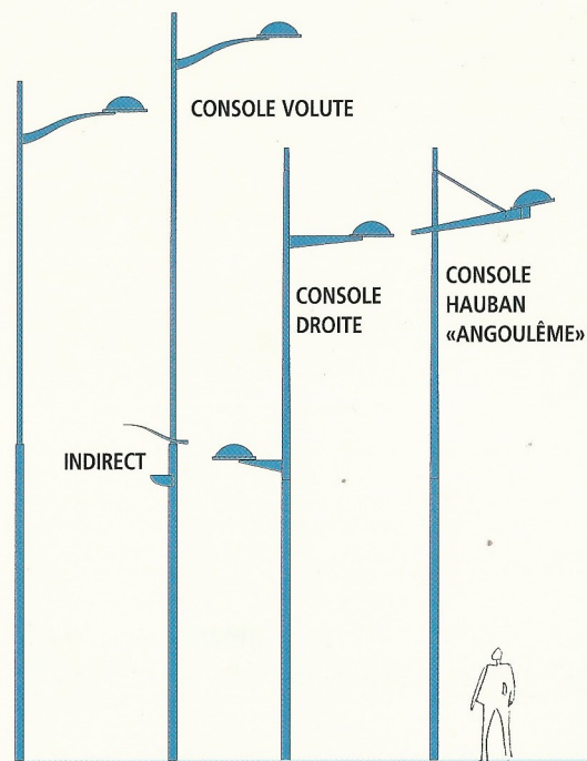
4 ensembles (mât rétreint, cylindrocônique) Hauteurs de 8,5 à 10 mètres
