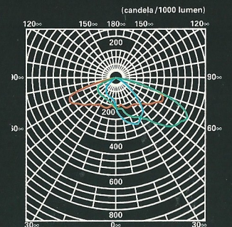
Jihem G 1XMac 2 «Antenna» 250W
