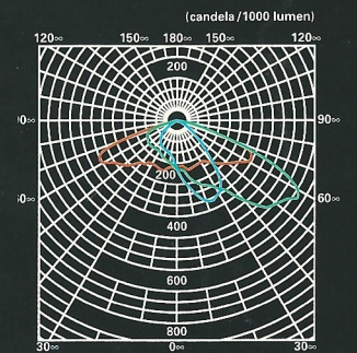
Jihem G 1XMac 2 «Antenna» 150W
