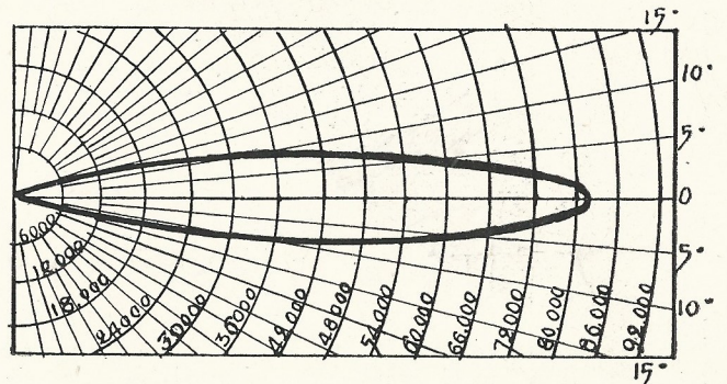
Courbe photométrique
