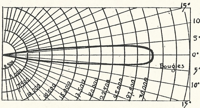
Courbe photométrique
